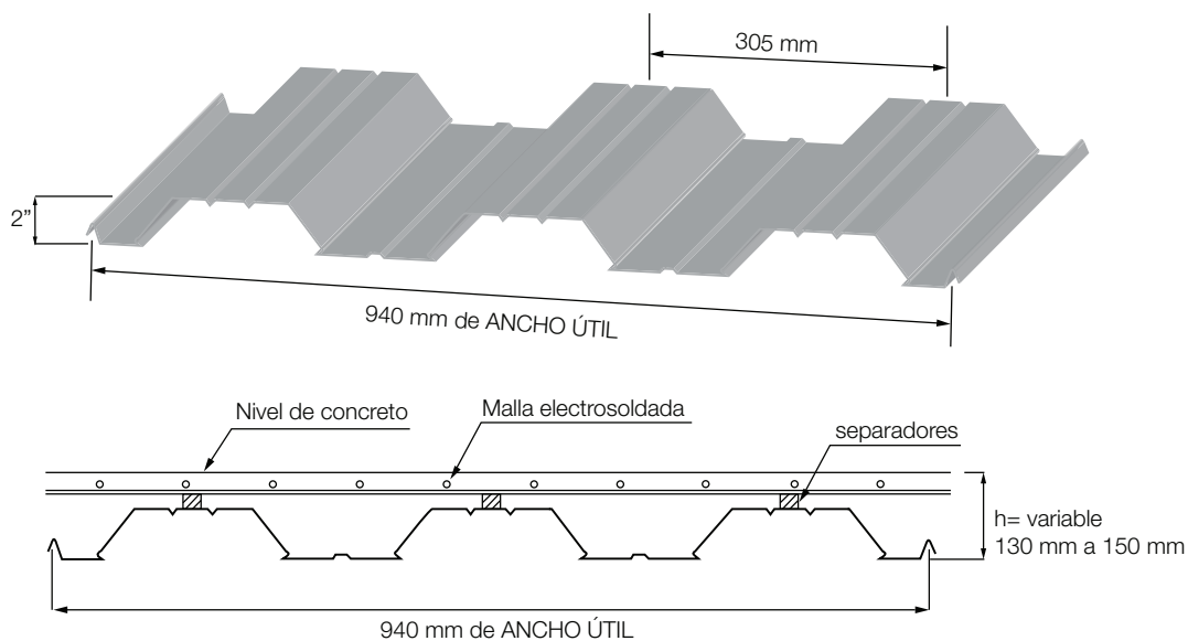
GEOMETRIA DEL METALDECK 2"
